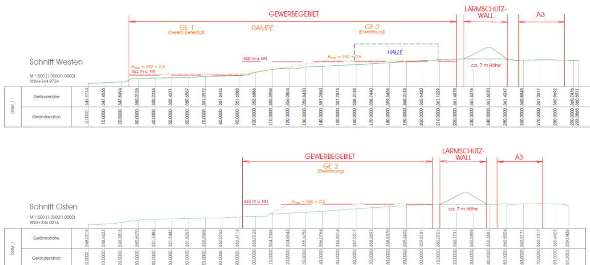
Geländeschnitte (Nord – Süd) auf Grundlage des DGM1-Rasters, unmaßstäblich
